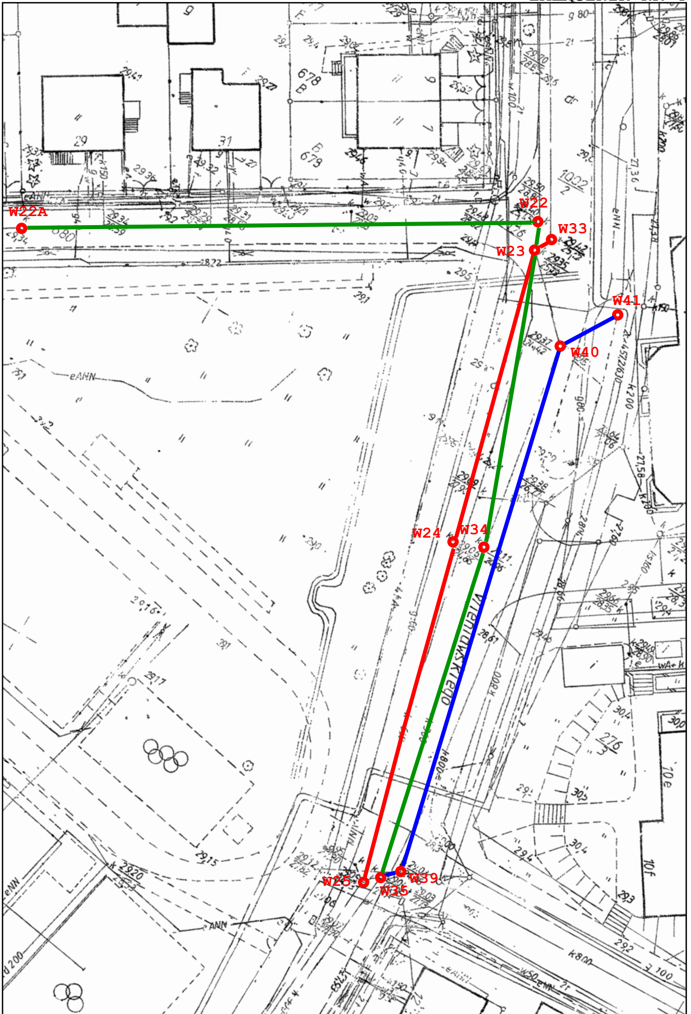
— SIEĆ KANALIZACYJNA DO REMONTU; DN300 — SIEĆ KANALIZACYJNA DO REMONTU; DN400 — SIEĆ KANALIZACYJNA DO REMONTU; DN600 SKALA 1:500
