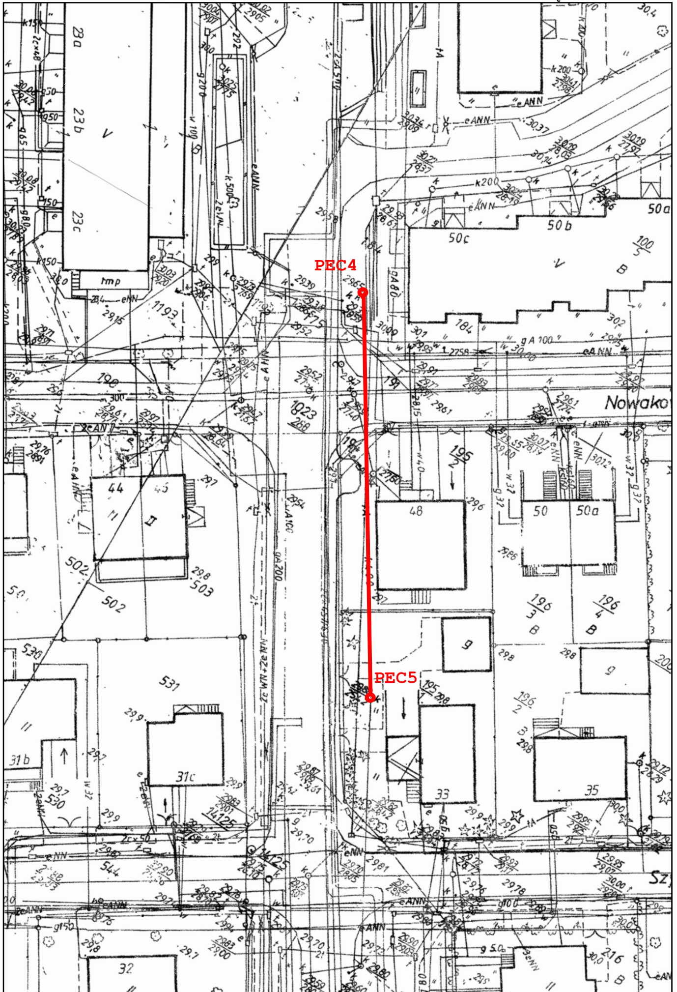
— SIEĆ KANALIZACYJNA DO REMONTU; DN400
