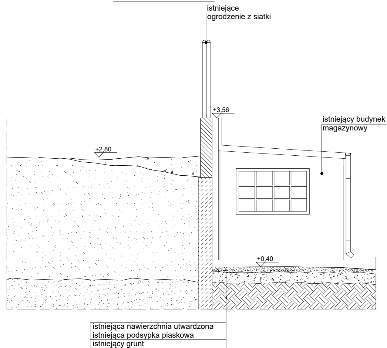
PRZEKRÓJ NR 4
