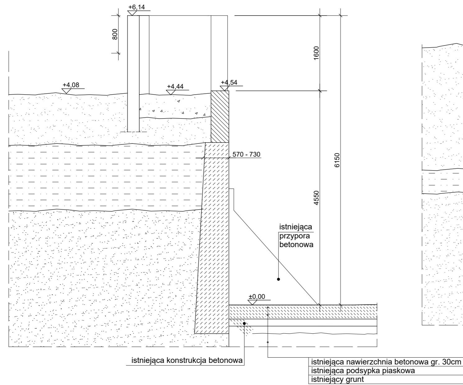
PRZEKRÓJ NR 4
