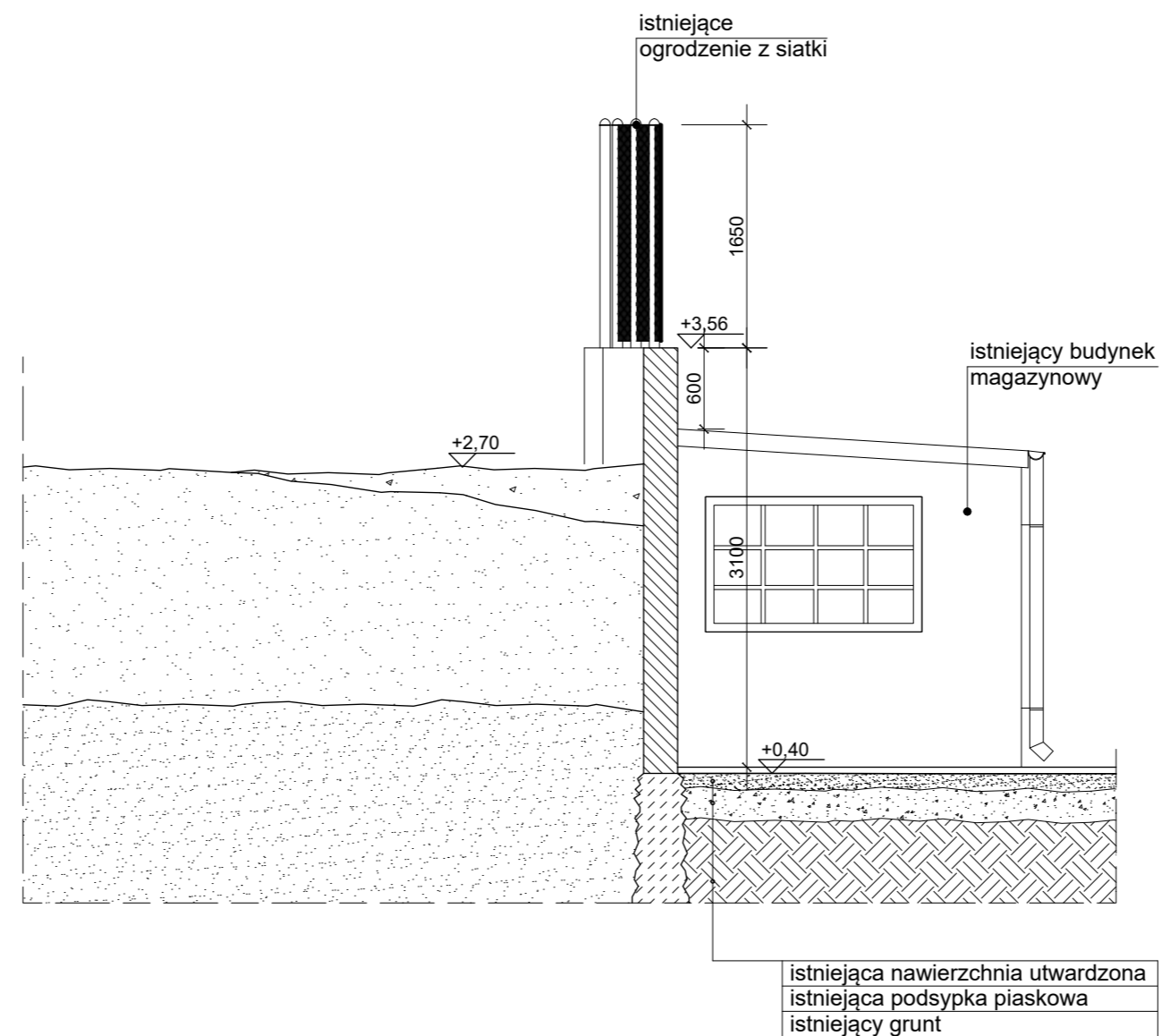
PRZEKRÓJ NR 5
