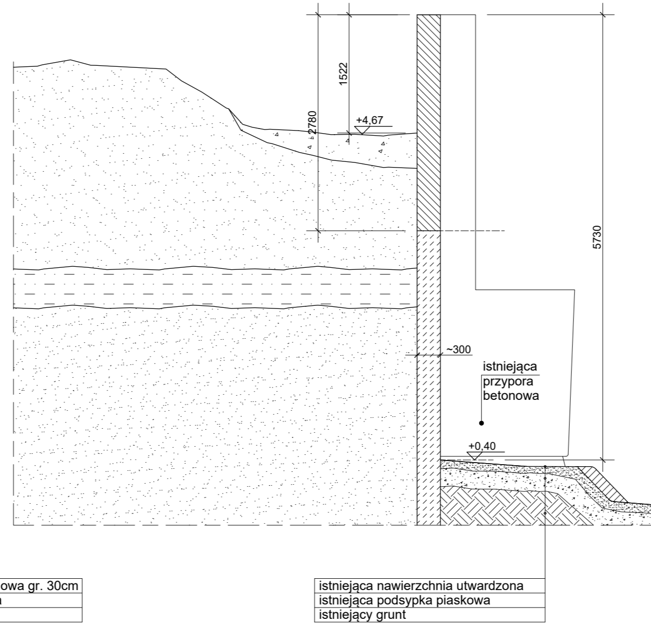
PRZEKRÓJ NR 5
