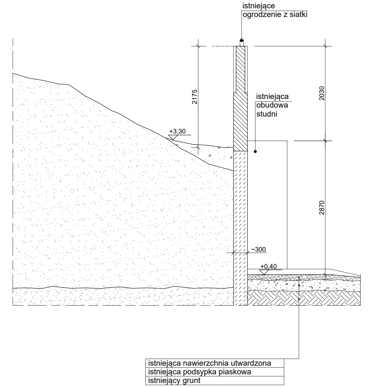
PRZEKRÓJ NR 3
